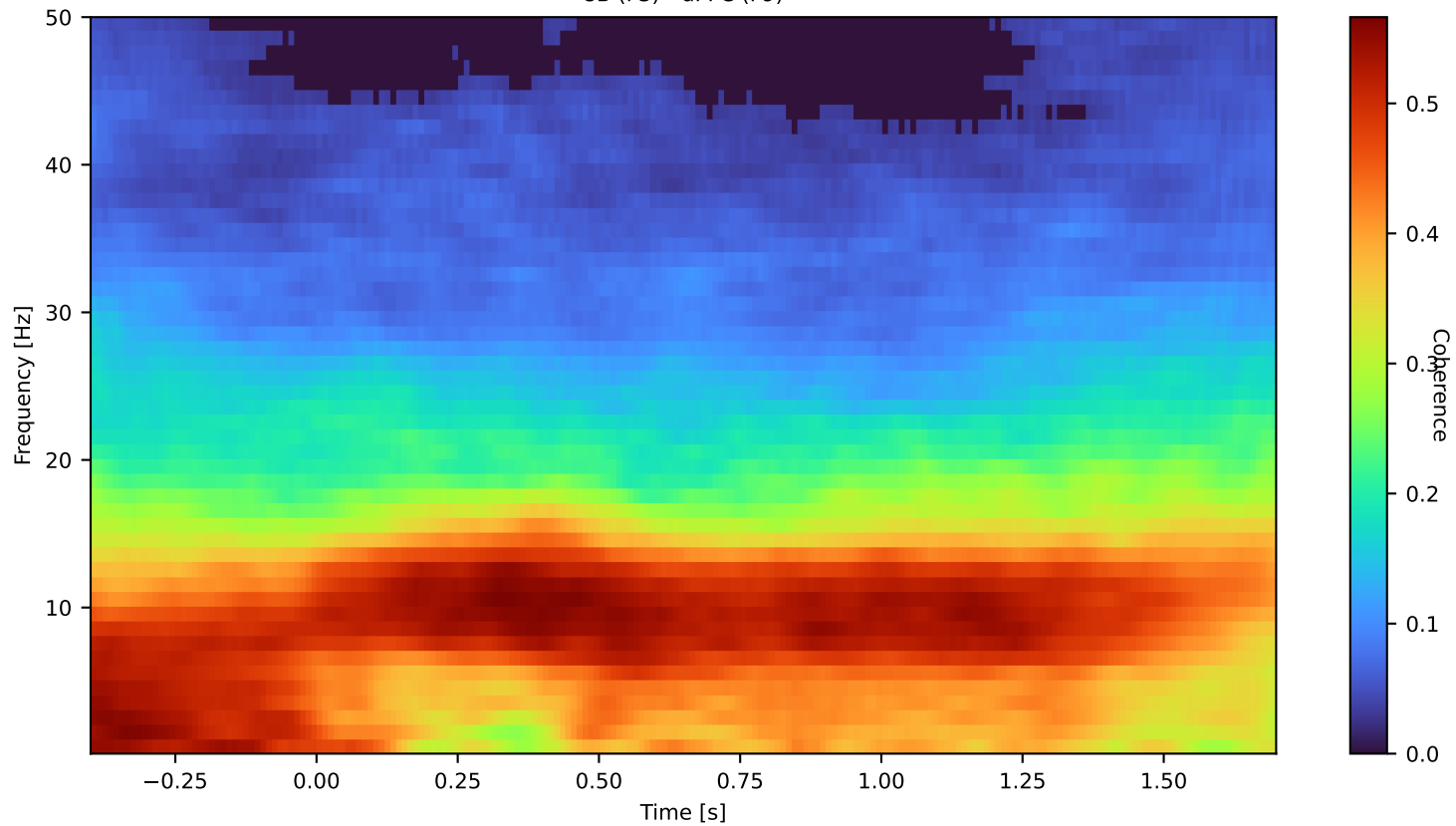
8B (F3) - dPFC (F9)
